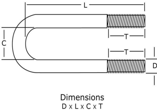
U-Bolt (round Bend)
